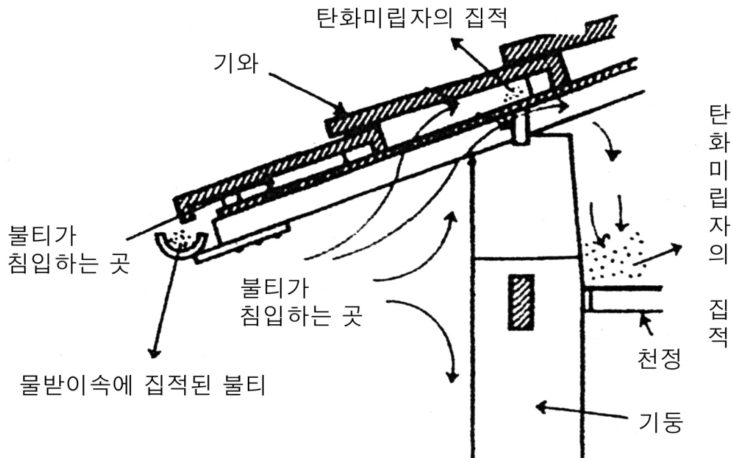
[그림 1-112] 처마 속으로 침입하는 불티와 탄화물의 집적장소
